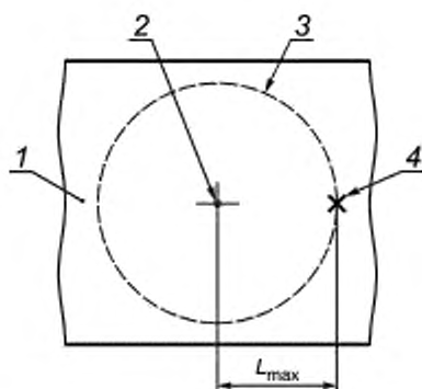
1 — фрагмент охраняемой конструкции; 2 — точка размещения чувствительного элемента извещателя; 3 — граница охраняемой зоны; 4 — место нанесения разрушающего воздействия; L_{\max} — максимальная дальность действия извещателя
