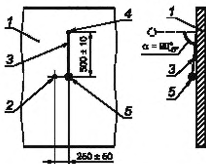
1 — фрагмент строительной конструкции; 2 — точка размещения чувствительного элемента извещателя; 3 — нить подвеса испытательного шара; 4 — точка крепления нити подвеса испытательного шара на поверхности охраняемой конструкции; 5 — испытательный шар
