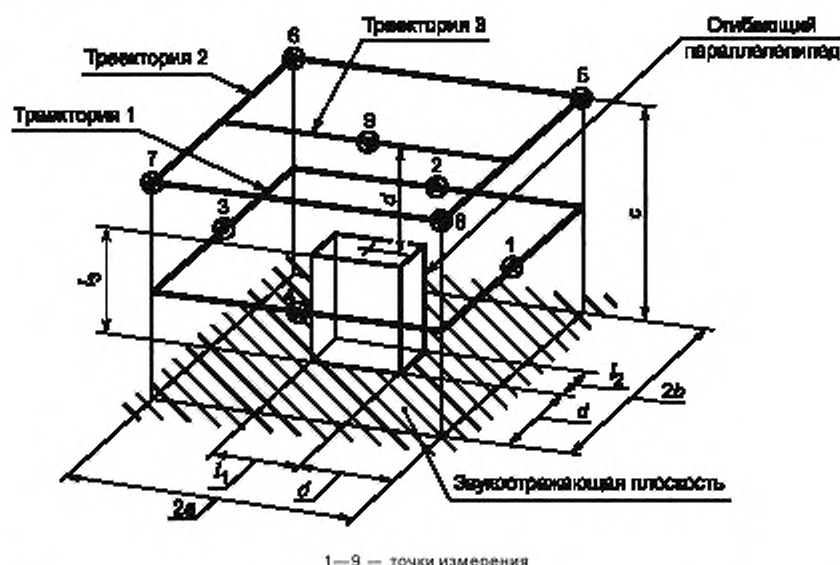
Рисунок 1 — Пример измерительной поверхности и положений (траекторий) микрофонов
