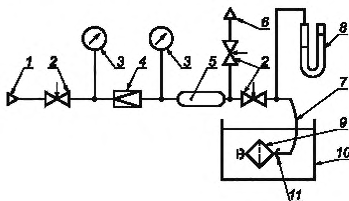
1 — подвод воздуха под давлением; 2 — вентиль; 3 — манометр; 4 — редуктор; 5 — ресивер; 6 — выпуск излишка воздуха в атмосферу; 7 — трубопровод гибкий (шланг); 8 — пьезометр; 9 — испытуемый фильтрующий элемент; 10 — ванна; 11 — заглушка фильтрующего элемента
