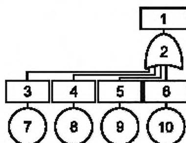
Рисунок 2 — Представление последовательной системы в виде ДН
