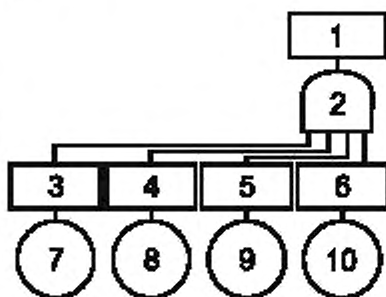
Рисунок 3 — Представление параллельной системы в виде ДН
