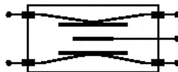
Рисунок 4д — Многосекционный проходной конденсатор
