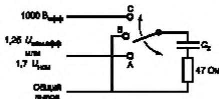
Сх — испытуемый конденсатор; U_{ном.эфф} — номинальное пульсирующее напряжение; U_{ном} — номинальное напряжение
