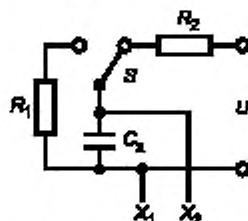
Сх — испытуемый конденсатор; R_1 — резистор, ограничивающий ток (разрядный); R_2 — резистор, ограничивающий ток (зарядный); S — переключающее устройство; U — испытательное напряжение; X_1 , X_2 — выводы для подключения осциллографа для регистрации максимальной скорости изменения напряжения
