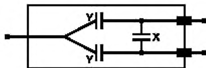
Рисунок 5b — Шунтирующий конденсатор, соединенный по схеме треугольника
