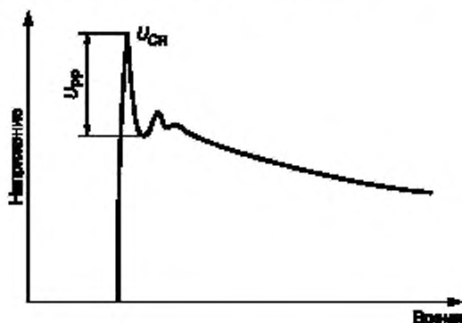
Рисунок 6 — Форма импульса
