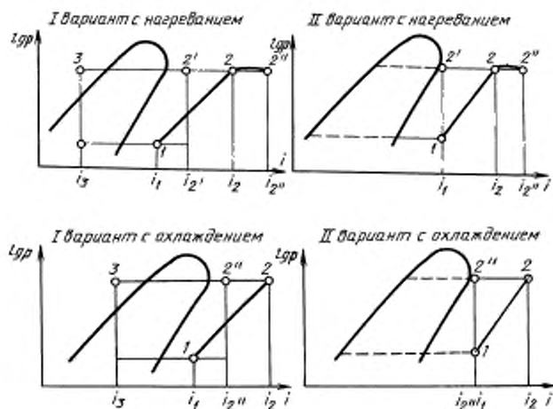
Точки рабочего цикла компрессора:
