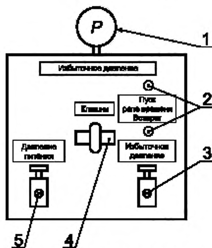
1 — манометр; 2 — реле времени; 3 — редуктор избыточного давления; 4 — пневматический цилиндр управления клешней; 5 — редуктор давления питания
