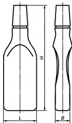
Бутылка БТ III-1-26 Рисунок А.26
