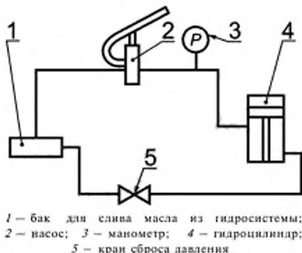
Рисунок 6 — Принципиальная схема пресса для испытания тары на сжатие
