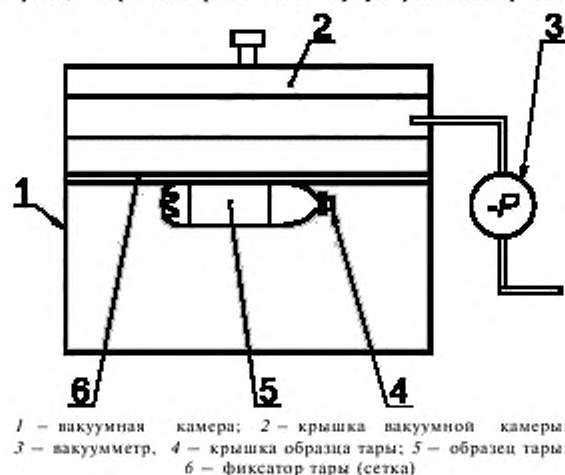
Рисунок 4 — Принципиальная схема испытания тары на герметичность укупоривания
