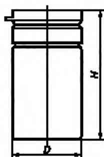
Банка БН 1-2-5 Рисунок А.5
