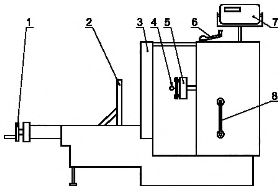
1 — устройство прижима тары; 2 — подвижный упор; 3 — неподвижный упор; 4 — серва; 5 — датчик усилий; 6 — рукоятка привода гидронасоса; 7 — цифровой вольтметр; 8 — рукоятка подъема гидроцилиндра
