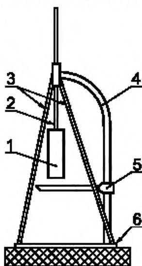
Рисунок 5 — Внешний вид стенда для испытания тары на удар при свободном падении
