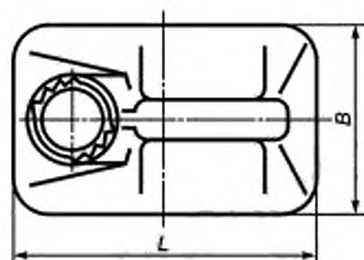
Канистра КН I-1-28 Рисунок А.28
