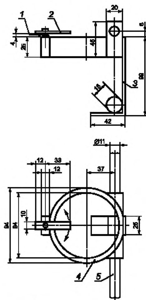
Рисунок 2 — Разливочное устройство
