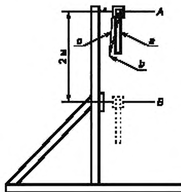
Рисунок А.1 — Испытание на механический удар
