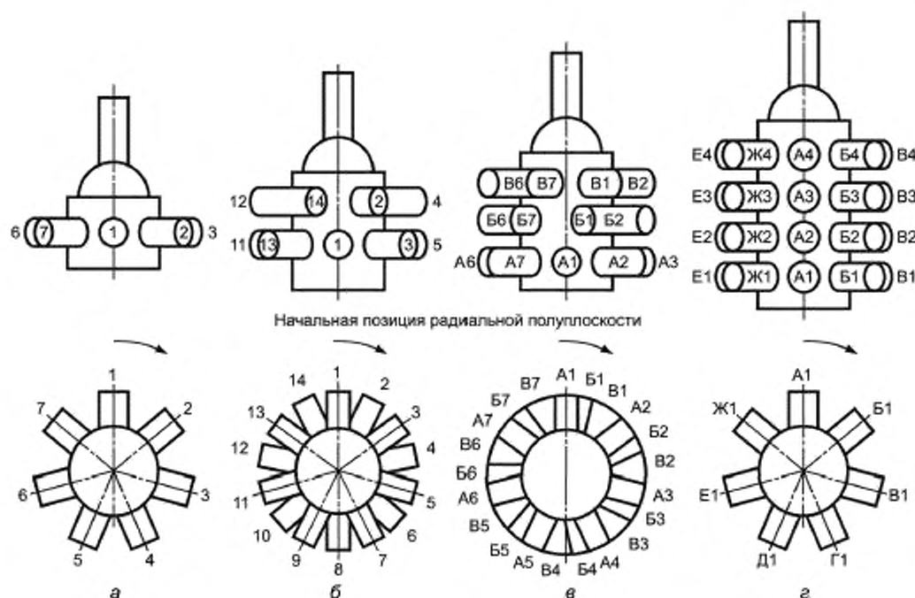
Рисунок 5 — Нумерация цилиндров поршневых двигателей с радиальным расположением цилиндров
