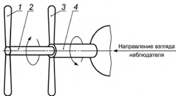
1, 3 — винт; 2 — внутренний вал, 4 — наружный вал
