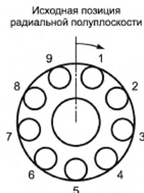
Рисунок 6 — Порядок нумерации узлов ГТД
