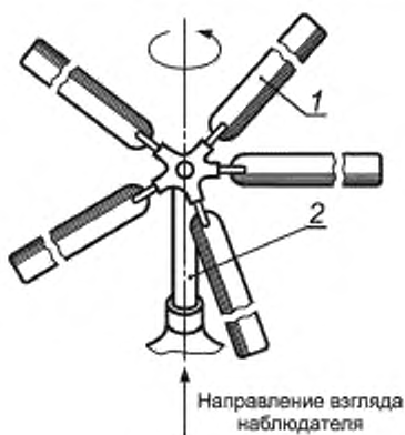
1 — винт; 2 — вал
