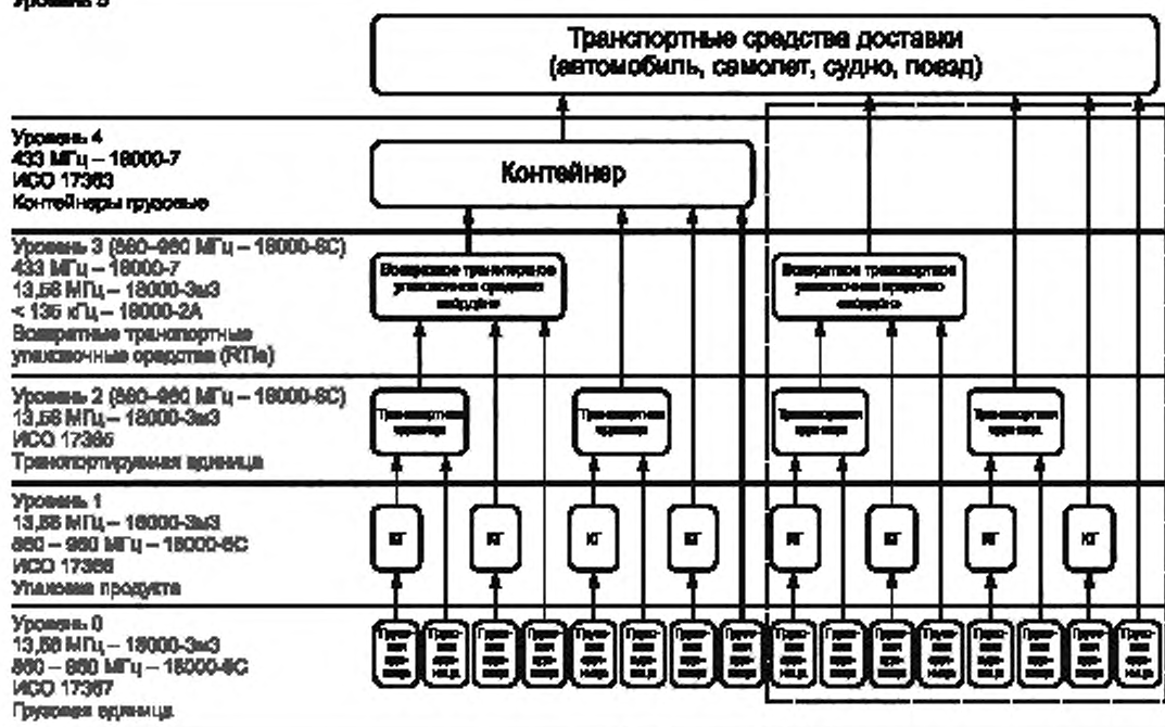
Рисунок 1 — Схематическая модель цепи поставок
