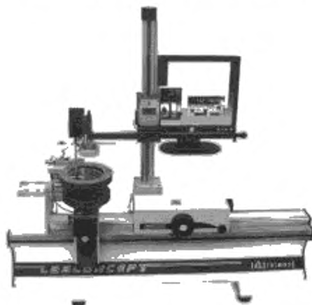
Рисунок Д.1 — Горизонтальный длиномер LabConcept 500
