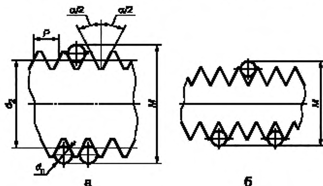
Рисунок 4 — Метод трех проволоочек
