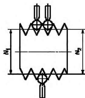
Рисунок 8 — Измерение среднего диаметра калибров-пробок на ДИП
