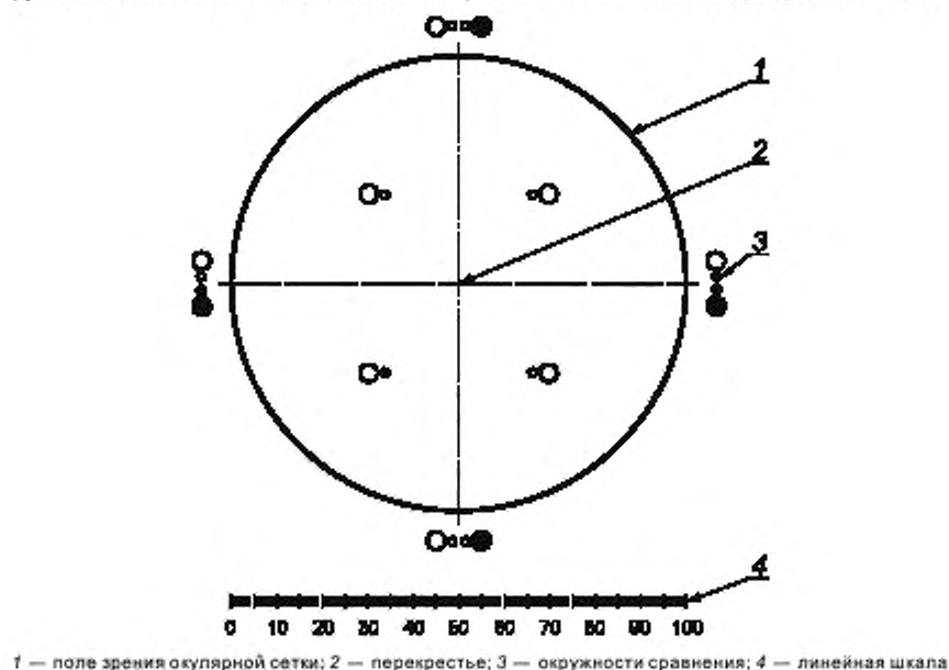
Рисунок Г.1 — Окулярная сетка с окружностями
