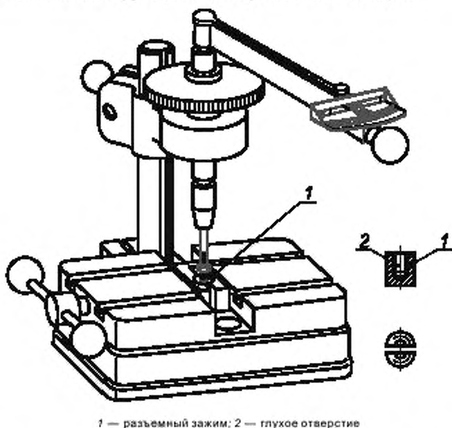
Рисунок 6 — Устройство для определения разрушающего крутящего момента M_B (6.2.5)
