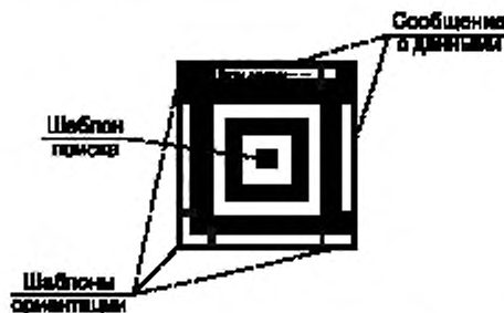
Рисунок А.2 — Структура символа Aztec Rune
