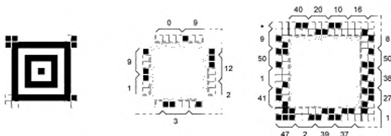
Рисунок G.1 — Последовательность построения символа Aztec Code
