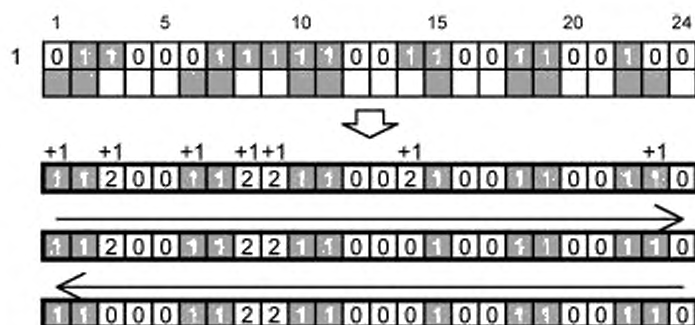
Рисунок С.3 — Последовательность и результаты сканирования строки 2
