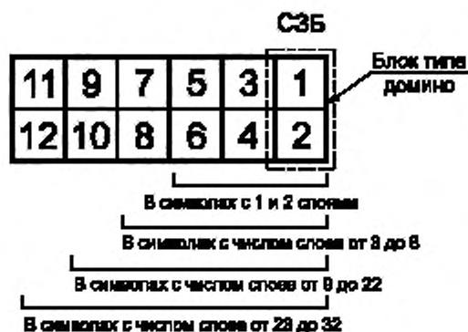
Рисунок 4 — Типовая структура знака в символе 2)
