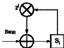
Рисунок В.2 — Схема генерирования значения синдромов
