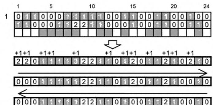
Рисунок С.4 — Последовательность и результаты сканирования строки 3
