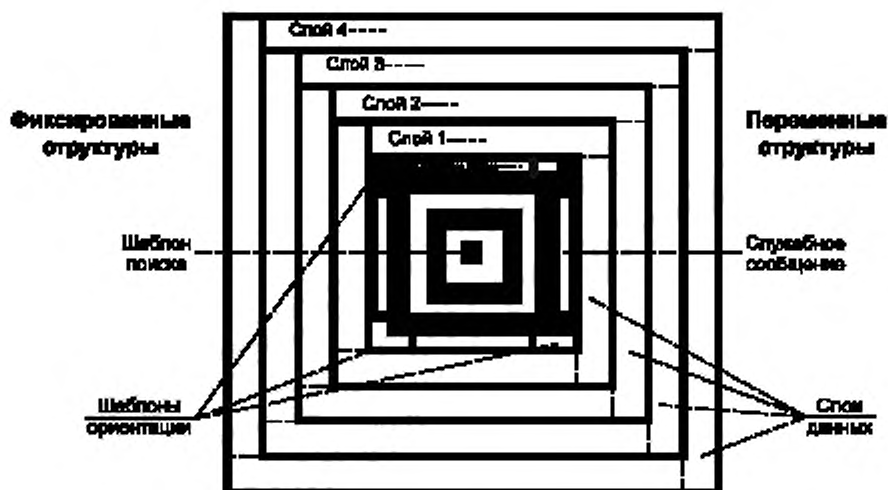
Рисунок 2 — Структура компактного символа Aztec Code
