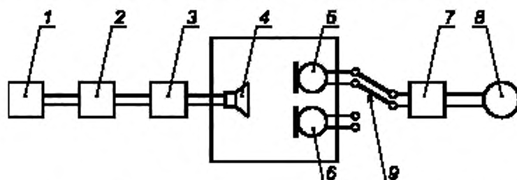
1 — генератор белого шума (5.1.2); 2 — 1/3-октавный фильтр (5.2.1); 3 — усилитель мощности (5.3.1); 4 — громкоговоритель (5.6.1); 5 — испытуемый микрофон, 6 — рабочий измерительный микрофон, отградуированный по свободному полю (5.5.2); 7 — микрофонный усилитель (5.3.2); 8 — вольтметр (5.4.2); 9 — переключатель
