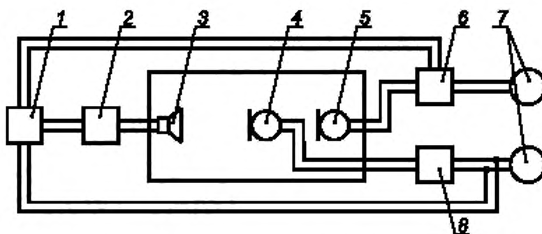
1 — установка для автоматической записи частотной характеристики (5.9.1); 2 — усилитель мощности (5.3.1); 3 — громкоговоритель (5.6.1); 4 — испытуемый микрофон; 5 — рабочий измерительный микрофон, отградуированный по свободному полю (5.5.2); 6 — установка для стабилизации звукового давления (5.9.3); 7 — вольтметр (5.4.1); 8 — микрофонный усилитель (5.3.2.)
