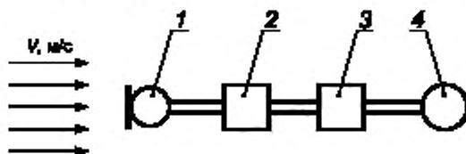
1 — испытуемый микрофон; 2 — микрофонный усилитель (5.3.2); 3 — 1/3-октавный фильтр (5.2.1); 4 — вольтметр (5.4.2)
