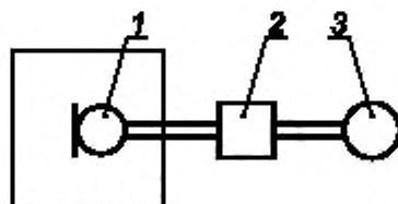
1 — испытуемый микрофон; 2 — измерительный усилитель (5.3.3); 3 — вольтметр (5.4.2)
