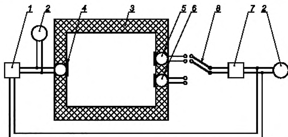
1 — установка для автоматической записи частотной характеристики (5.9.1); 2 — вольтметр (5.4.1); 3 — установка (5.9.6); 4 — излучатель; 5 — испытываемый микрофон; 6 — рабочий измерительный микрофон в соответствии с требованиями 5.5.2, отградуированный по давлению; 7 — микрофонный усилитель (5.3.2); 8 — переключатель
