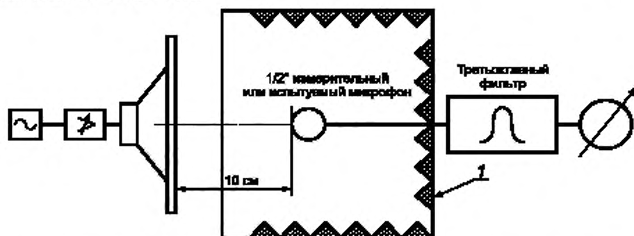
Рисунок ДБ.4 — Испытательная установка для измерения чувствительности по звуковому полю
