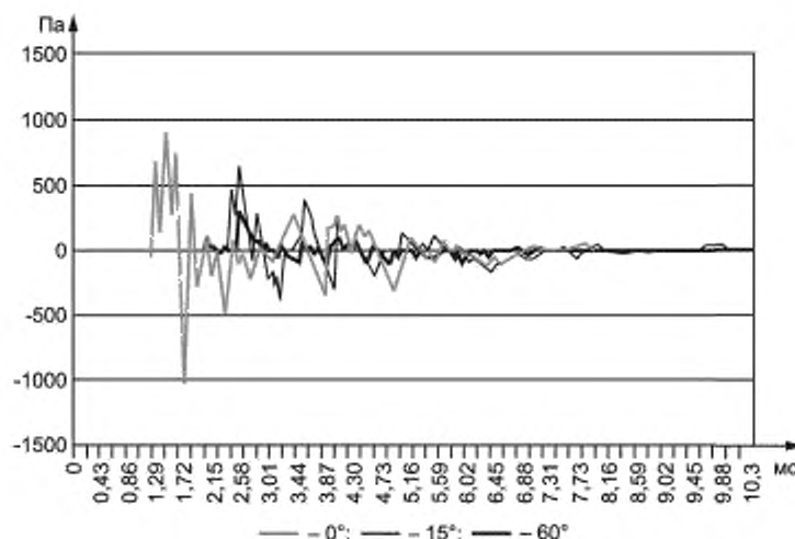
Рисунок А.1 — Зависимость звукового давления от времени для углов 0°, 15° и 60° для ствола длиной 0,67 м с полным чоком при дробовом снаряде массой 24 г с дульной скоростью 400 м/с
