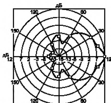
Рисунок А.5 — Диаграмма направленности D(\alpha) уровня углового распределения энергии источника для октавной полосы 1 кГц, построенная с помощью интерполяции кубическим сплайном и L_Q , рассчитанным по формуле (14)
