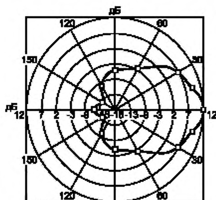
Рисунок А.4 — Диаграмма направленности D(\alpha) уровня углового распределения энергии источника для октавной полосы 1 кГц, построенная с помощью интерполяции кубическим сплайном и L_{Q^*} , рассчитанным по формуле (15)
