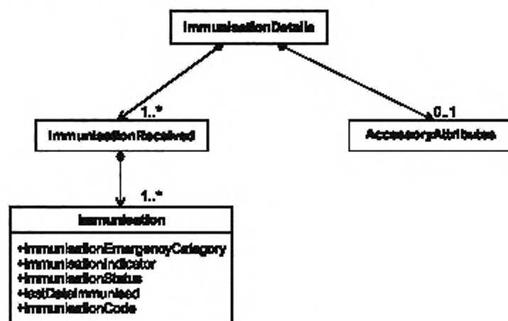
Рисунок 4 — Структура класса информационных объектов «ImmunizationDetails»
