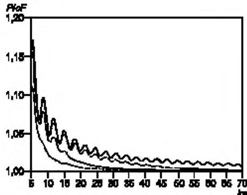
Рисунок Е.2 — Зависимость P/cF от ka для четырех различных псевдотрапецевидных амплитудных распределений: для \epsilon = 0 (поршень) (сплошная кривая), \epsilon = 0,1 (штриховая), \epsilon = 0,25 (точечная), \epsilon = 0,6 (штрихпунктирная)
