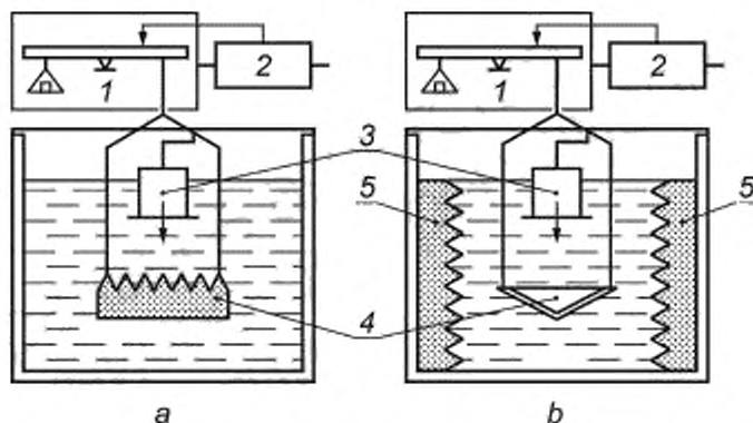
Рисунок F.5 — Компонка Е с поглощающей (а) и вогнутой отражающей (б) мишенями:
