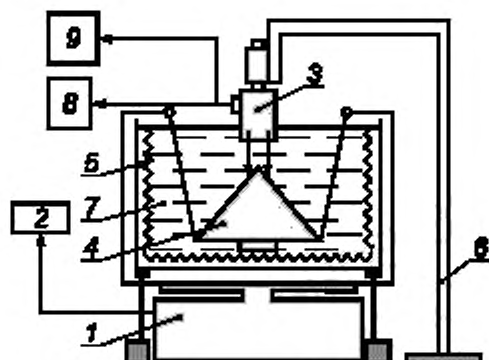
Рисунок F.2 — Компонка В с выпуклой отражающей мишенью:
