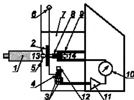
Рисунок F.7 — Компонетка F с поглощающей мишенью:
