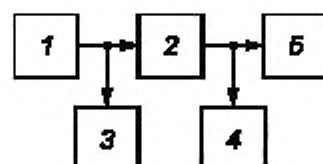
Рисунок 4 — Схема измерения коэффициента нелинейных искажений
