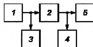
Рисунок 3 — Схема измерения неравномерности амплитудно-частотной характеристики
