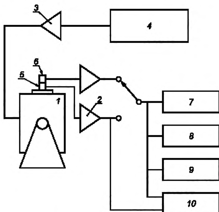
1 — вибростенд; 2 — усилители; 3 — усилитель мощности; 4 — генератор сигнала; 5 — эталонный преобразователь; 6 — калибруемый преобразователь; 7 — вольтметр; 8 — измеритель коэффициента гармоник; 9 — осциллограф (необязательный элемент); 10 — измеритель фазового сдвига (необязательный элемент)
