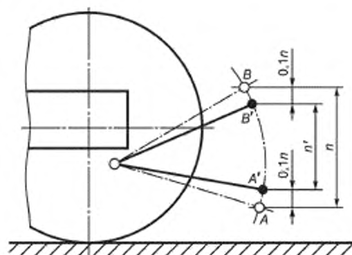
Рисунок 1 — Диапазон перемещения
