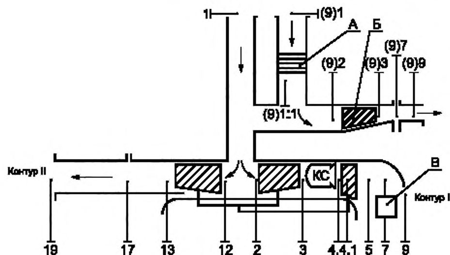
Рисунок 6 — Схема нумерации сечений вспомогательного силового блока с двумя раздельными входными потоками
