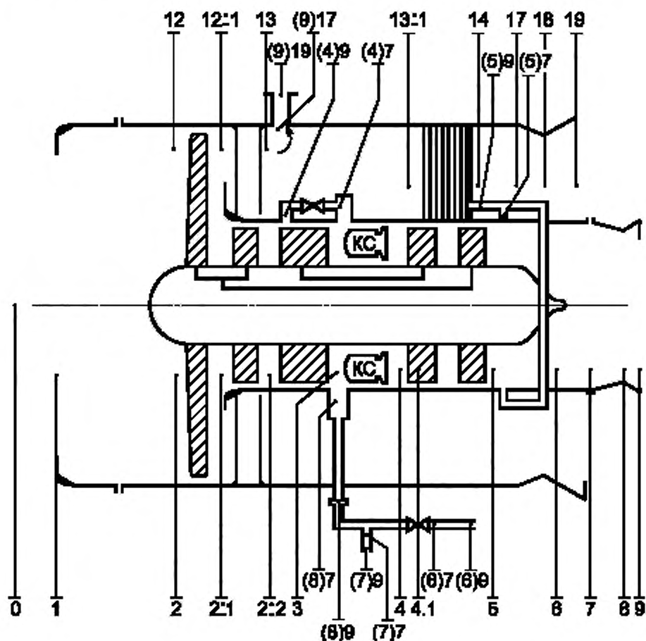
Рисунок 8 — Схема нумерации контрольных сечений для ТРДД без смешения контуров с системами отборов, перепуска и регенерации тепла. Нумерация сечений — см. таблицу 3
