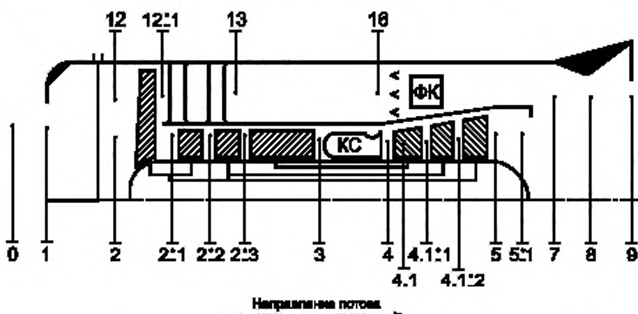
Рисунок 2 — Схема контрольных сечений для двигателей ТРДД со смешением контуров и общим соплом
