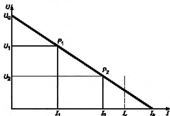
Рисунок 2 — Нагрузочные характеристики генераторов тока
