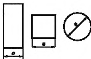
Рисунок ДА.1 — Формы и размеры отверстия
