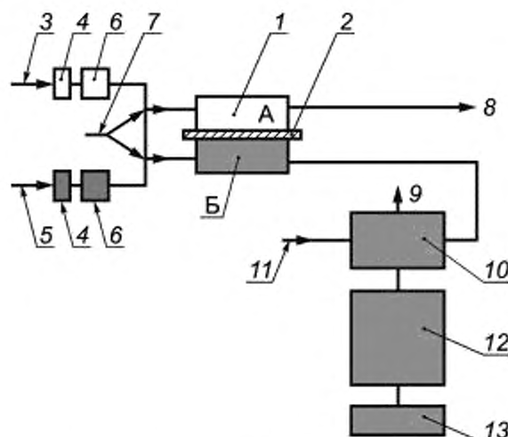
1 — диффузионная ячейка с камерами А и Б; 2 — образец; 3 — вход газа для испытания; 4 — устройство для кондиционирования газа; 5 — вход газа-носителя; 6 — расходомер; 7 — трехходовой кран; 8 — выход газа для испытания (или газа-носителя при продувке); 9 — выход газа-носителя; 10 — дозирующая петля; 11 — вход газа-носителя для хроматографа; 12 — хроматографическая колонка; 13 — детектор по теплопроводности (ТПД) или пламенно-ионизационный детектор (ПИД)
