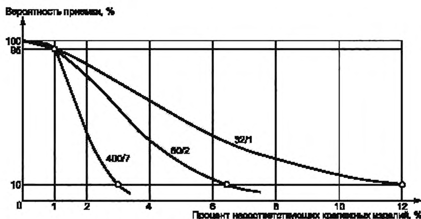
Пример — AQL = 1, планы выборочного контроля 32/1, 80/2 и 400/7
