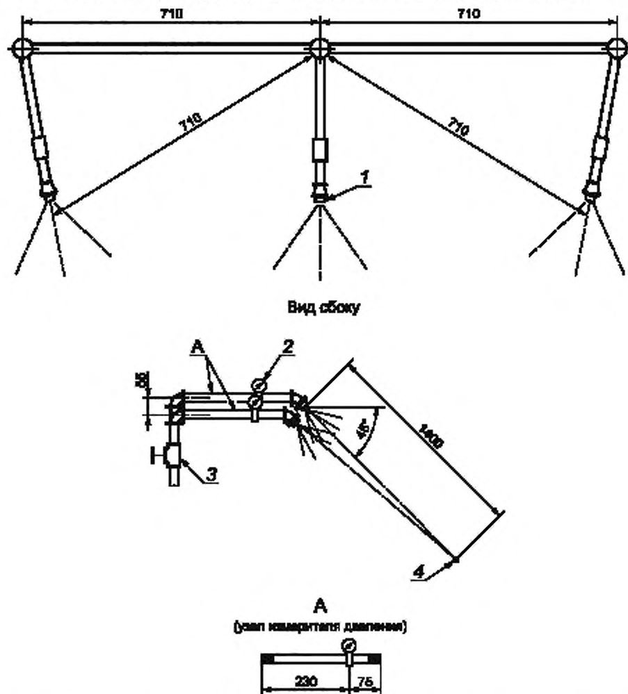
1 — распылительная головка (см. рисунок В.2); 2 — измеритель давления для каждой распылительной головки в отдельности; 3 — регулятор давления для каждой распылительной головки в отдельности, 4 — центральная точка
