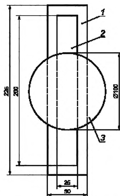
1 — опорная плита из оцинкованной или крашеной стали толщиной 1,5—3,5 мм; 2 — испытуемый образец закрепляют на опорной плите, используя клеящие вещества и технологические методы, предложенные изготовителем, 3 — цилиндрический груз массой 18 кг
