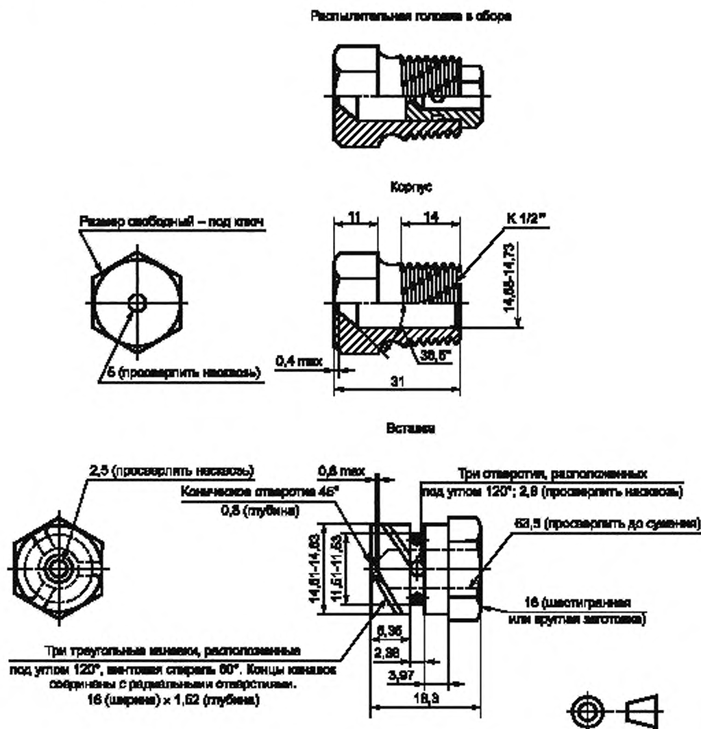
Рисунок В.2 — Распылительная головка
