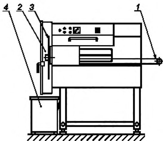
1 — питающий транспортер; 2 — дверца камеры для нарезания; 3 — серводвижное/многоsegmentное лезвие; 4 — контейнер
