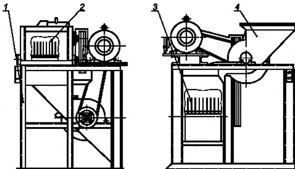
1 — станция; 2 — первый ножовой барабан с дисковыми ножами; 3 — второй ножовой барабан с дисковыми ножами; 4 — загрузочная камера
