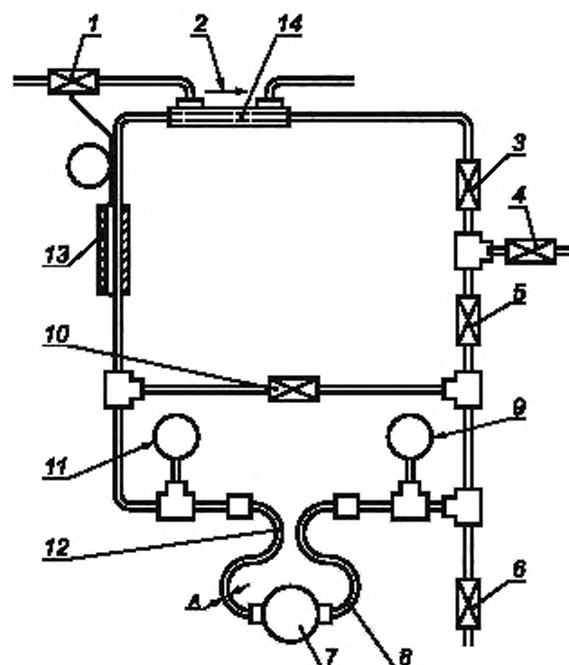
1 — терморегулирующий водяной клапан; 2 — охлаждающая вода; 3 — устройство управления всасыванием; 4 — впускной клапан; 5 — устройство управления давлением нагнетания; 6 — выпускной клапан; 7 — мотор-компрессор ; 8 — линия давления нагнетания; 9 — нагнетание; 10 — клапан для выравнивания давления; 11 — всасывание; 12 — линия всасывания; 13 — датчик терморегулятора; 14 — теплообменник
