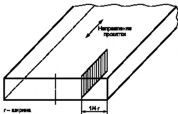
Рисунок 4 — Образец от листа толщиной не более 25 мм
