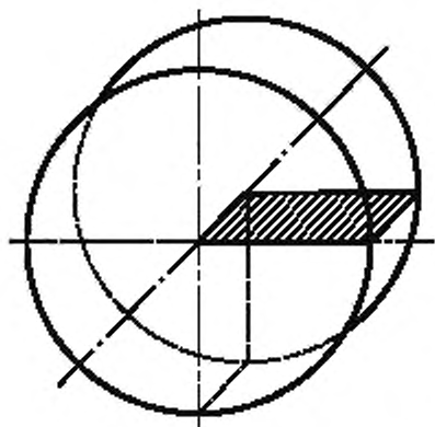
Рисунок 2 — Образец от прутка или заготовки диаметром или длиной стороны свыше 25 до 40 мм включительно
