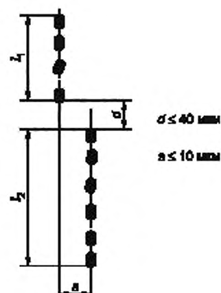
Рисунок 9 — Включения типа В
