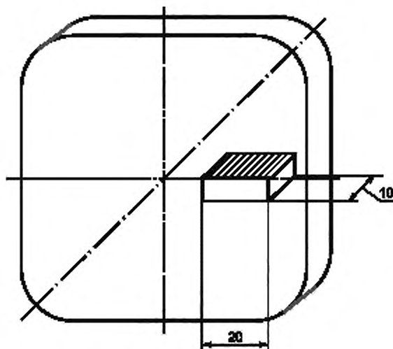
Рисунок 1 — Образец от прутка или заготовки диаметром или длиной стороны свыше 40 мм
