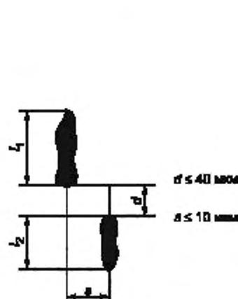
Рисунок 8 — Включения типов А и С
