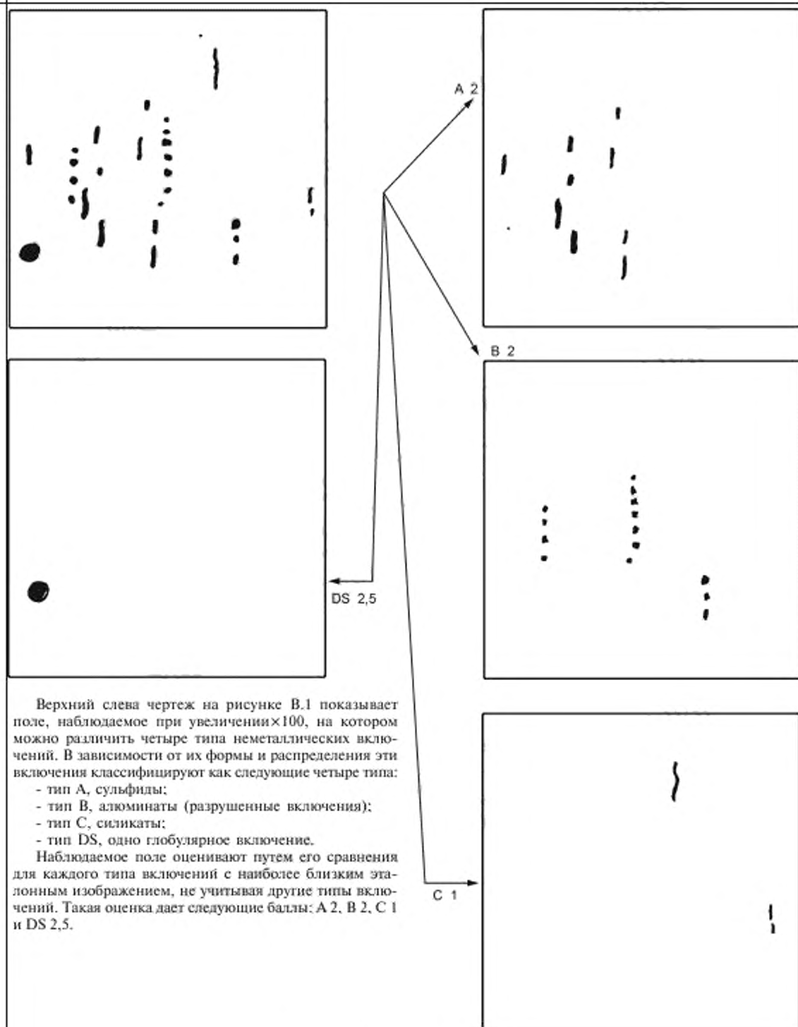
Рисунок В.1 — Оценка поля
