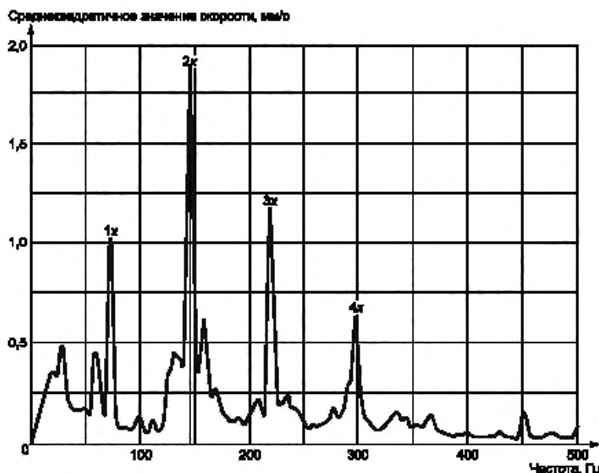
Рисунок 14 — Частотный спектр
