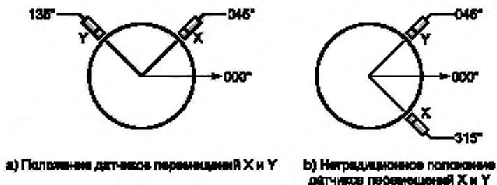
Рисунок D.9 — Обозначение датчиков перемещений бесконтактного типа
