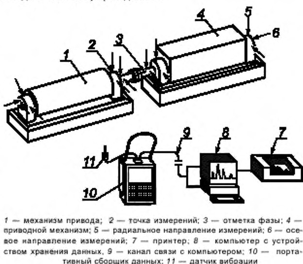
Рисунок 2 — Типичная переносная система контроля
