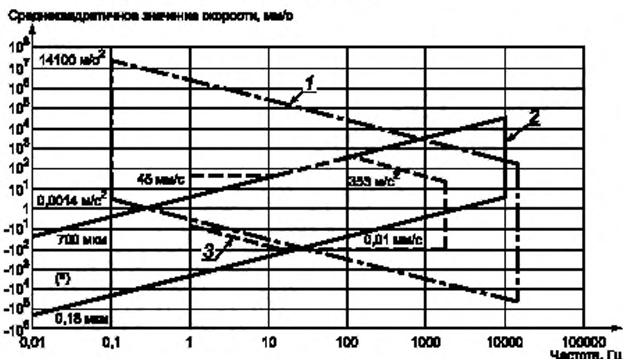
1 — пьезоэлектрический акселерометр; 2 — вихревой датчик; 3 — электрохимический датчик скорости
