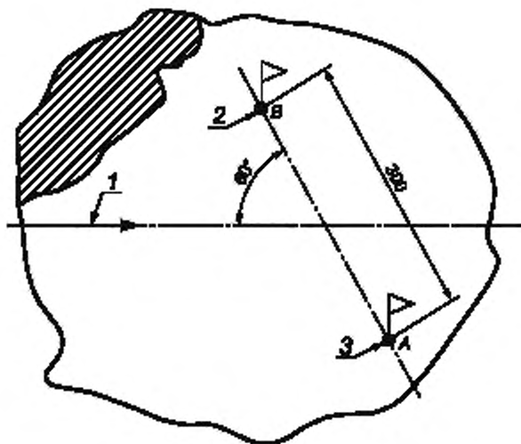
Рисунок В.3 — Испытание под парусом
