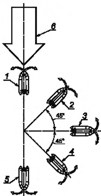
1 — курс против ветра; 2 — 45° в шквал; 3 — курс при боковом ветре. 4 — 45° по корме; 5 — курс по ветру 6 — истинный ветер
