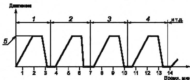
1 — отсек 1; 2 — отсек 2; 3 — отсек 1; 4 — отсек 2; 5 — проектное рабочее давление
