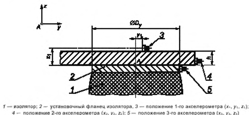
Рисунок 5 — Возможные положения акселерометра для измерений v_y
