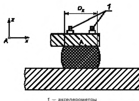
1 — акселерометры
