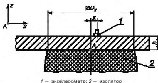
Рисунок 4 — Положение акселерометра для измерений v_z
