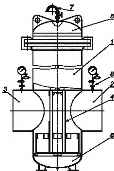
1 — корпус; 2, 3 — боковые патрубки входа и выхода нефти; 4 — фильтрующий элемент; 5 — крышка; 6 — днище с опорами; 7 — патрубков для контроля давления; 8 — патрубки для установки манометров
