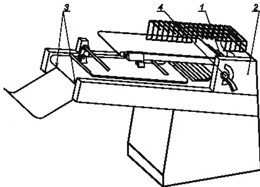
Рисунок 7 — Схема опасных зон тестовоформирующей машины 3-го типа
