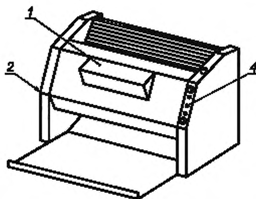
Рисунок 5 — Схема опасных зон тестоформирующей машины 1-го типа
