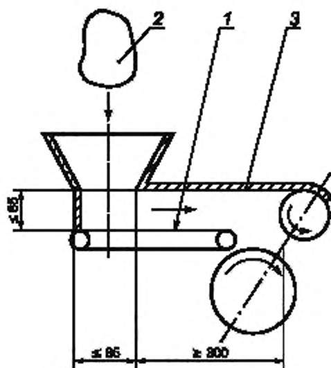
1 — лента, 2 — тестовая заготовка; 3 — кожух
