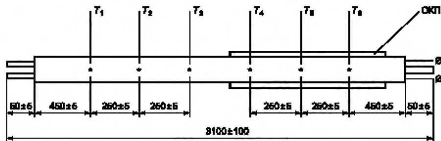
Рисунок 1 — Размещение термоэлектрических преобразователей
