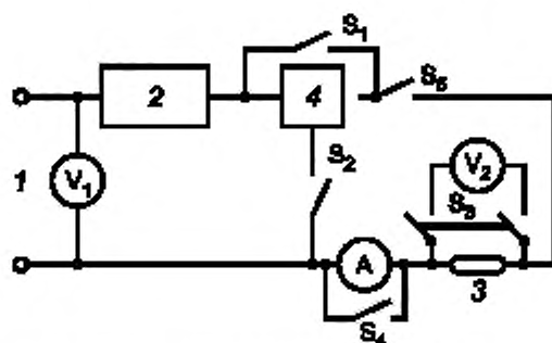
1 — синусоидальный источник питания; 2 — ДОО; 3 — лампа; 4 — 3У
