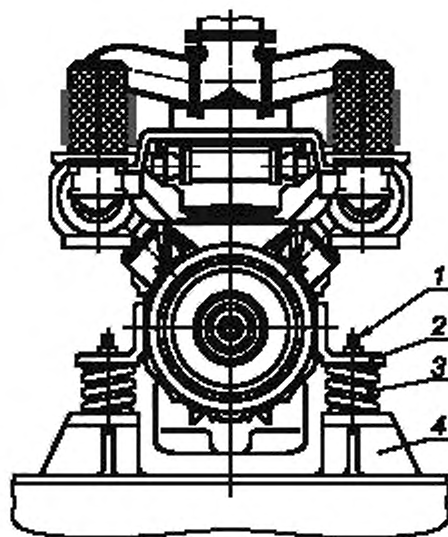
1 — акселерометр; 2 — опорная лапа; 3 — изолятор; 4 — основание
