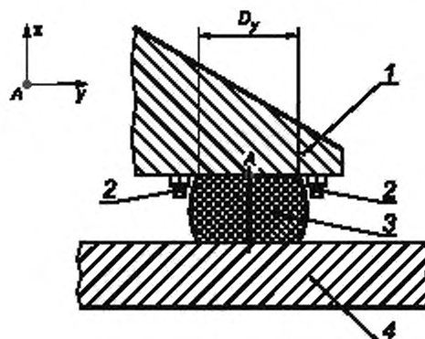
Рисунок 5 — Установка двух акселерометров для измерений v_z
