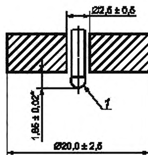
f — полусфера диаметром (1,575 \pm 0,025) мм
