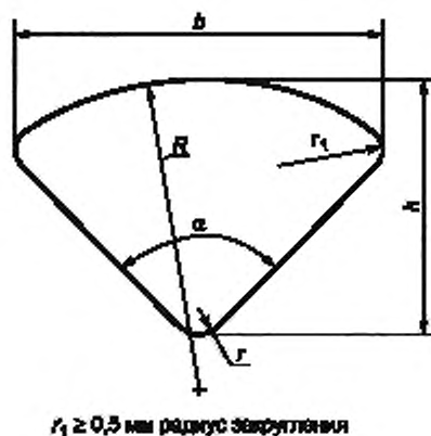
Рисунок А.2 — Конструкция секторных однопроволочных алюминиевых жил
