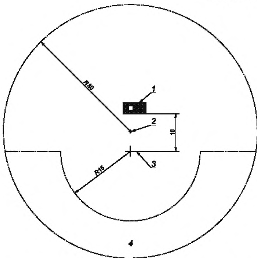
Рисунок В.1 — Открытая измерительная площадка
