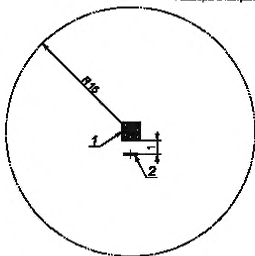
Рисунок D.1 — Открытая измерительная площадка
