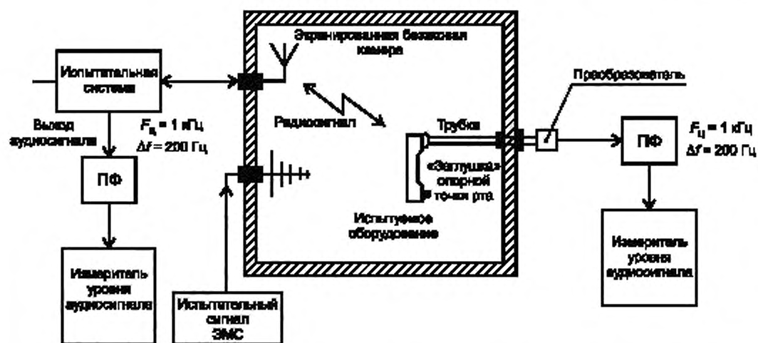
Рисунок 2 — Схема прохождения сигнала при испытаниях портативного оборудования
