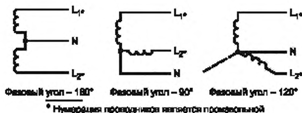
Рисунок 3 — Двухфазная трехпроводная система
