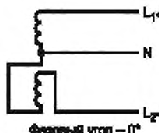
Рисунок 2 — Однофазная трехпроводная система
