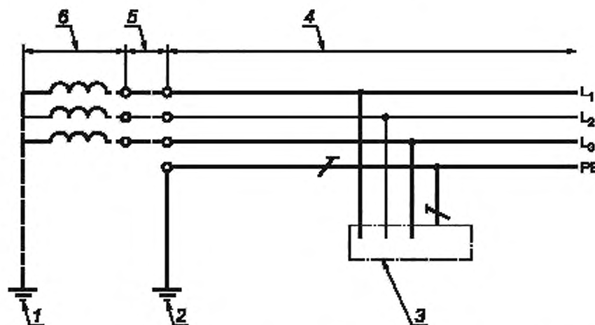
Рисунок 31F1 — Система TT трехфазная четырехпроводная с заземленным защитным проводником и нейтральным проводником во всей системе
