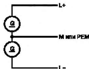
Рисунок 7 — Трехпроводная система
