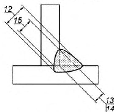
г) угловой шов с разными катетами Fillet weld with unequal legs Soudure d'angle asymétrique
