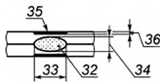
g) шов при точечной контактной сварке
