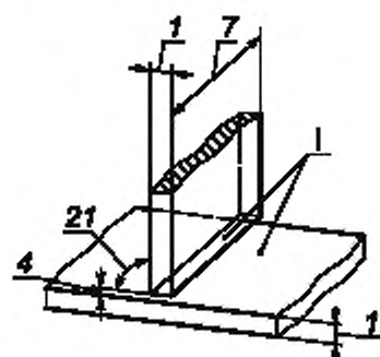
Рисунок 6 — Подготовка под сварку таврового соединения
