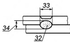
h) шов при рельефной сварке
