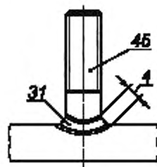
c) шов при приварке шпильки
