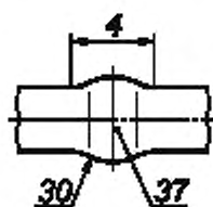
a) шов с гратом при стыковой сварке сопротивлением
