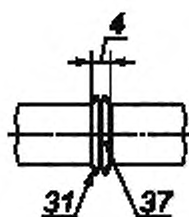
b) шов с гратом при стыковой сварке оплавлением или трением
