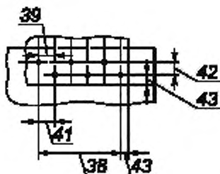
f) двойной ряд сварных точек, расположенных в шахматном порядке
