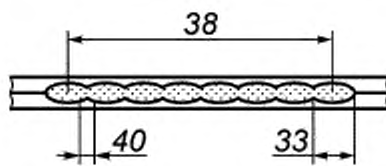
e) шов при шовной контактной сварке
