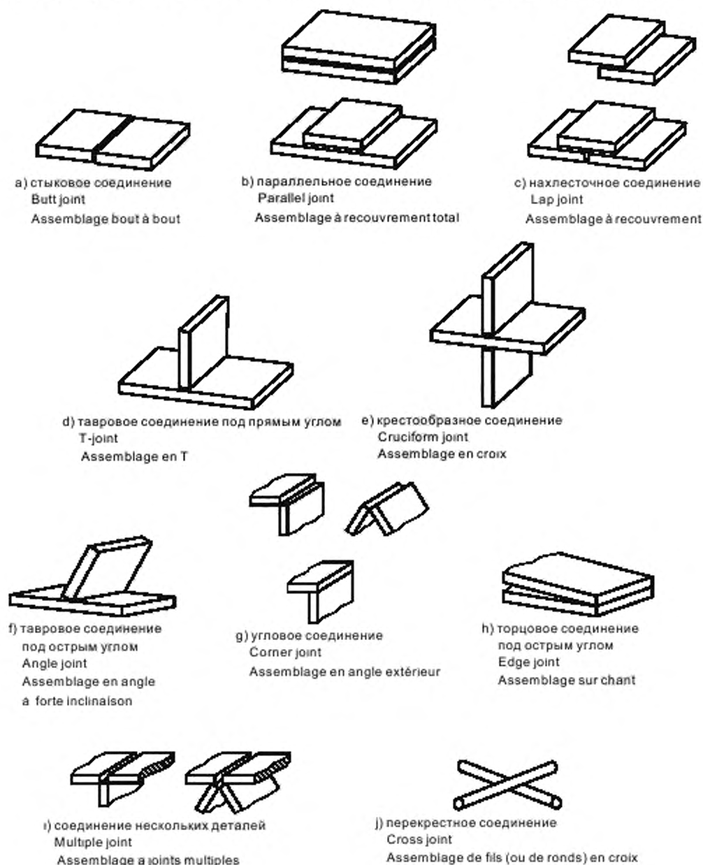
Рисунок 1 — Типы соединений
