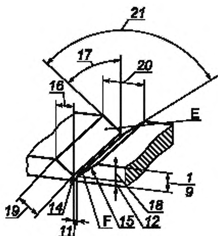
Рисунок 4 — Подготовка под сварку стыкового соединения с V-образным скосом кромок и с притуплением
