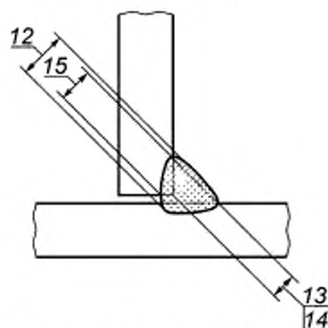
в) угловой шов с зазором Fillet weld with gap Soudure d'angle avec jeu
