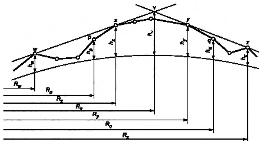
w — ближайшая точка предыдущего затеняющего препятствия; x — ближайшая к левому концу интервала точка рассматриваемого препятствия; y — ближайшая к правому концу интервала точка рассматриваемого препятствия; z — ближайшая точка следующего затеняющего препятствия; p — точка отметки высоты рельефа, предшествующая x; q — точка отметки высоты рельефа, следующая за y; v — точка пересечения касательных лучей, проведенных от соседних затеняющих препятствий
