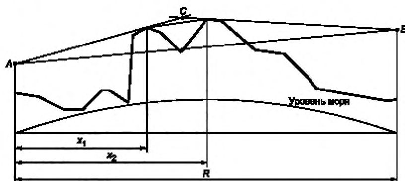
А — левая антенна; В — правая антенна; x_1 , x_2 — расстояния от левой антенны до препятствий, R — длина радиорелейного интервала
