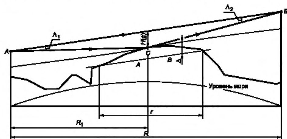
A — левая антенна; B — правая антенна; C — точка отражения; H(g) — просвет в точке отражения; A'B' — прямая, параллельная линии AB; r — расстояние между точками, в которых прямая A'B' пересекает неоднородность рельефа; R_1 — расстояние от левой антенны до точки отражения; R — длина трассы радиорелейного интервала
