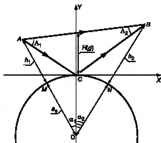
A — левая антенна; B — правая антенна; C — точка отражения; H(g) — просвет в точке отражения; a_0 — эквивалентный радиус Земли; h_1, h_2 — высота антенн ЦРПС над уровнем моря
