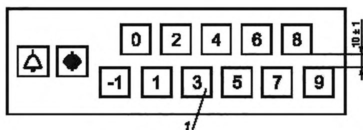
Рисунок В.3 — Пост управления в кабине при двухрядном горизонтальном расположении кнопок приказов
