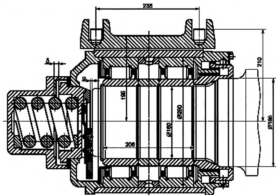
Рисунок Г.1 — Букса колесной пары тепловоза ТЭ3
