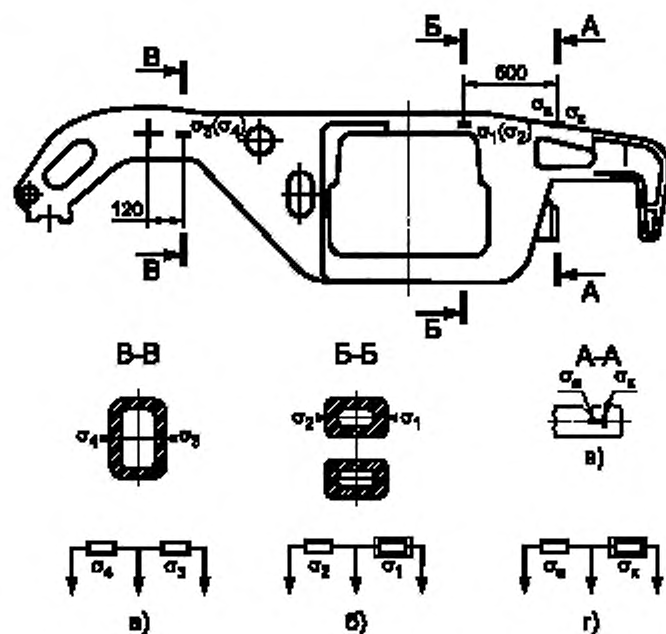
а) схема соединения датчиков в сечении В—В; б) схема соединения датчиков в сечении Б—Б; в) схема наклейки датчиков в сечении А—А; г) схема соединения датчиков в сечении А—А
