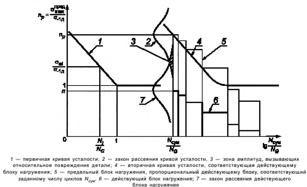
Рисунок 1 — График уравнения вторичной кривой усталости в относительных координатах
