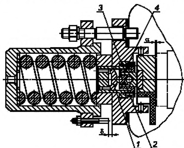
1 — мессдоза; 2 — промежуточная деталь; 3 — втулка; 4 — вспомогательная пружина
