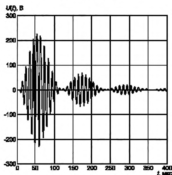
Рисунок 1 — Типичная форма радиоимпульса в антенне тиратронного передатчика ИФНС «Чайка»
