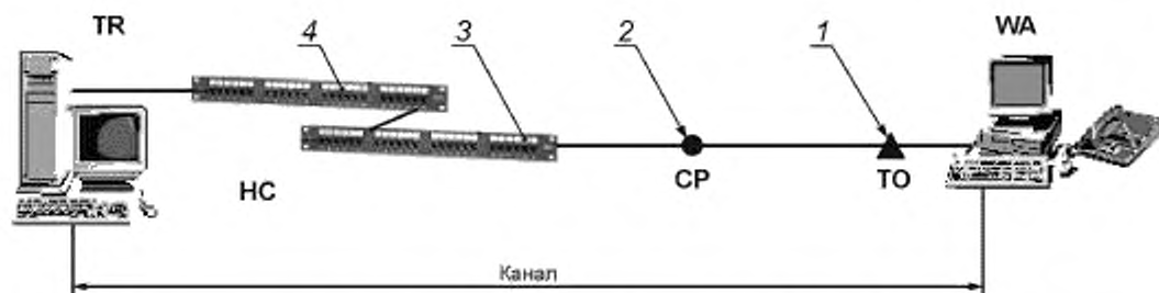
1 — коннектор телекоммуникационной или многопользовательской розетки (ТО или MuTOA), 2 — коннектор консолидационной точки (CP); 3 — коннектор первой единицы коммутационного оборудования в горизонтальном кроссе (HC); 4 — коннектор второй единицы коммутационного оборудования в горизонтальном кроссе (HC)
